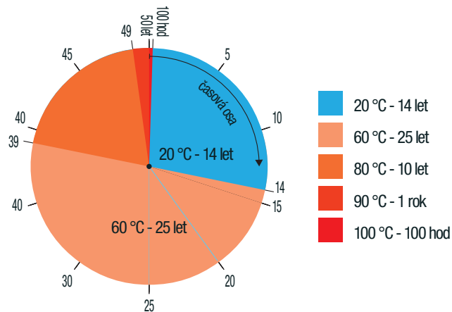
GRAF 4 - Graf životnosti trubek 50 let za současného působení teploty a času pro třídě použití 5 podle ISO 10508:2006 (E)
