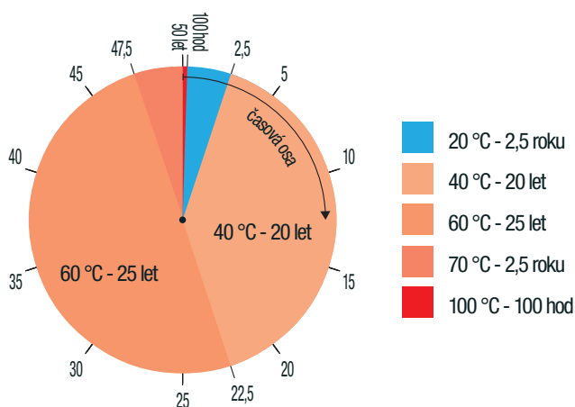
GRAF 3 - Graf životnosti trubek 50 let za současného působení teploty a času pro třídě použití 4 podle ISO 10508:2006 (E)
