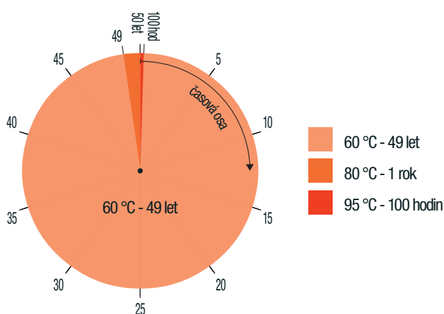
GRAF 1 - Graf životnosti trubek 50 let za současného působení teploty a času pro třídě použití 1 podle ISO 10508:2006 (E)
